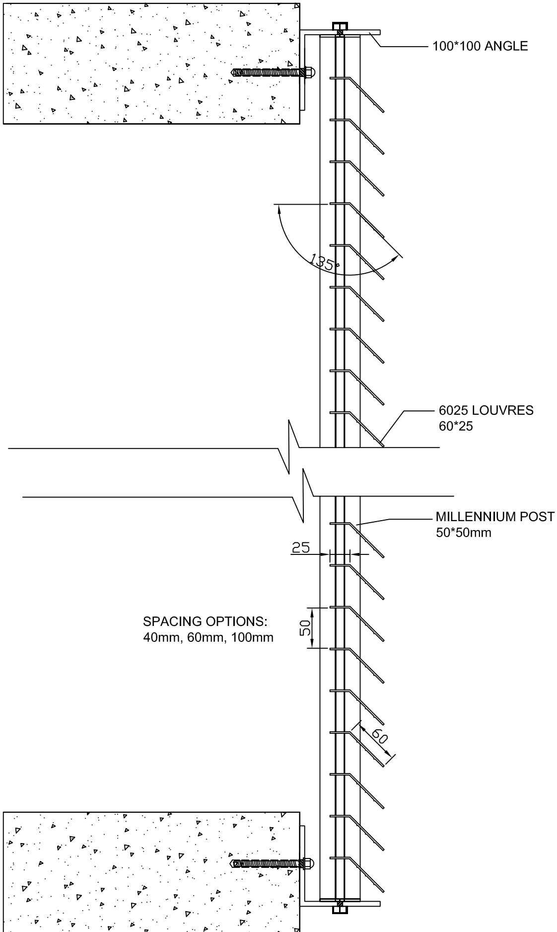
6025 LOUVRES ANGLE FACE-FIXED
